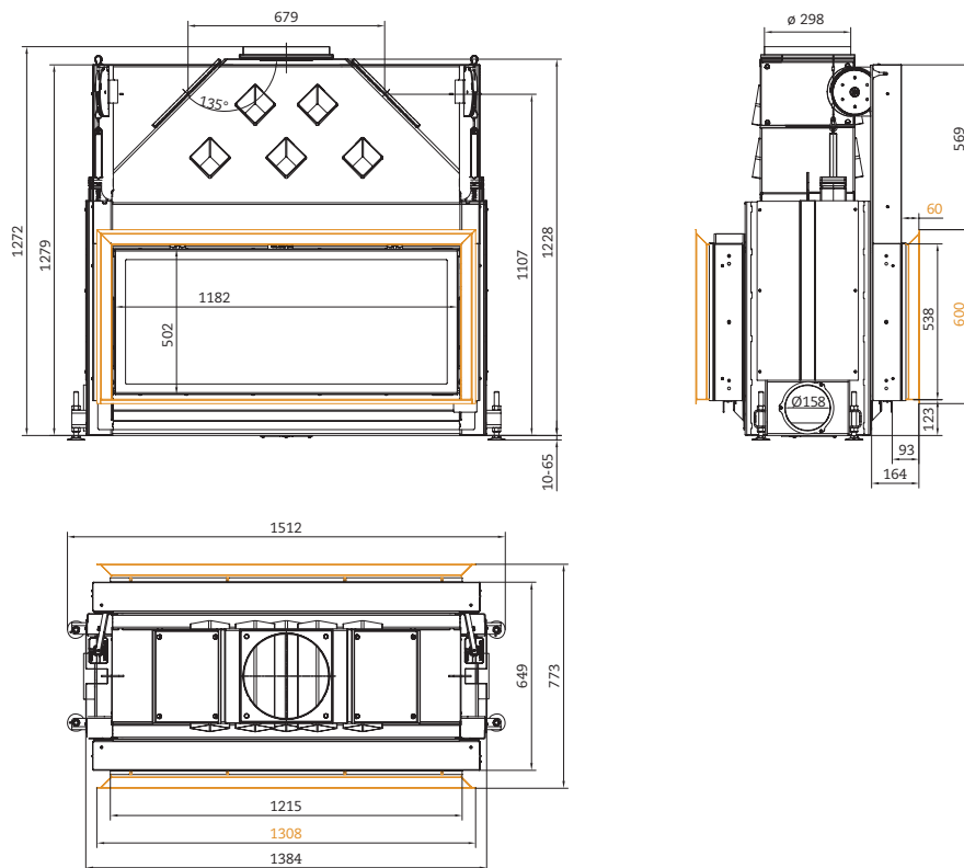
... Schiebetür / Kipptür mit Blendrahmen
