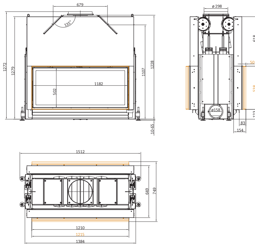
... Schiebetür / Schiebetür mit Anbaurahmen
